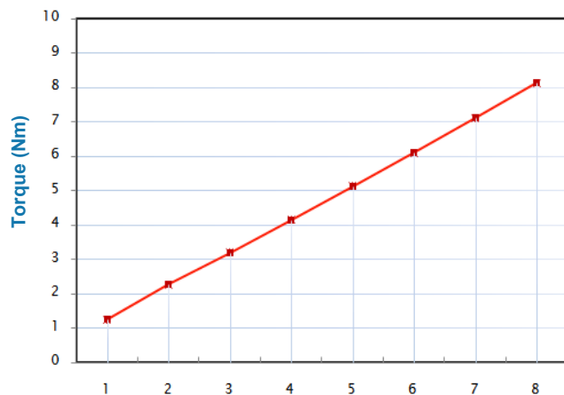
Input Torque
